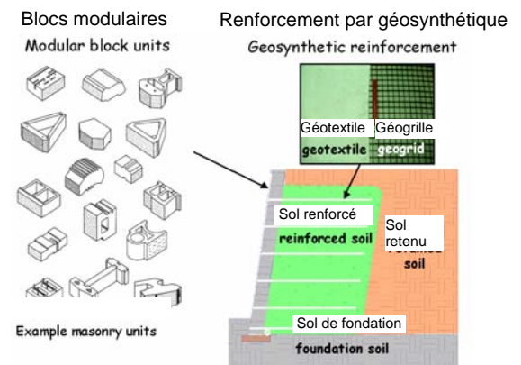
Exemples de blocs modulaires en béton
