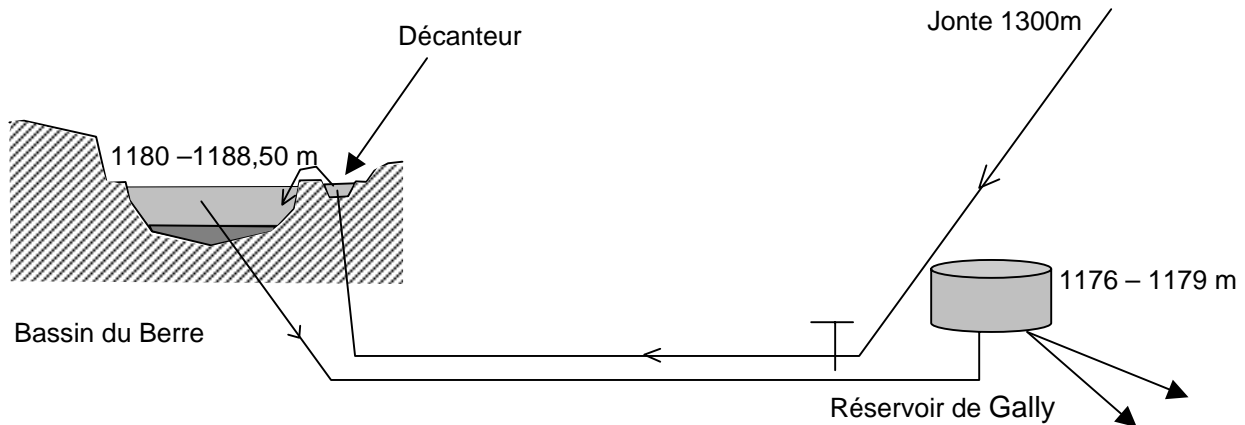
Figure 2. Coupe de l'aménagement
