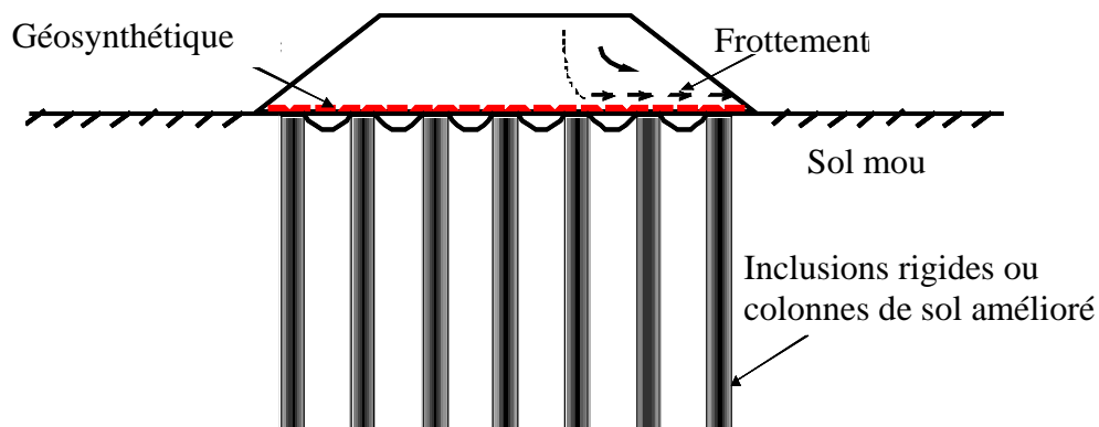
Renforcement par inclusions rigides et plate-forme de transfert de charge
