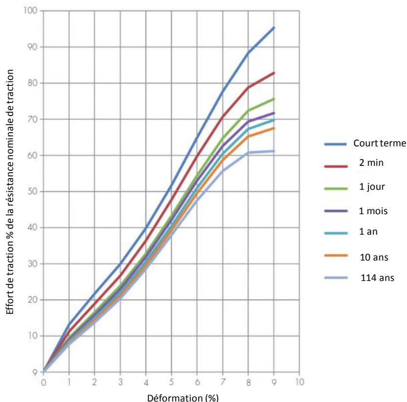
Figure 6. Courbes isochrones du géotextile de renforcement (température de référence 20°C)
