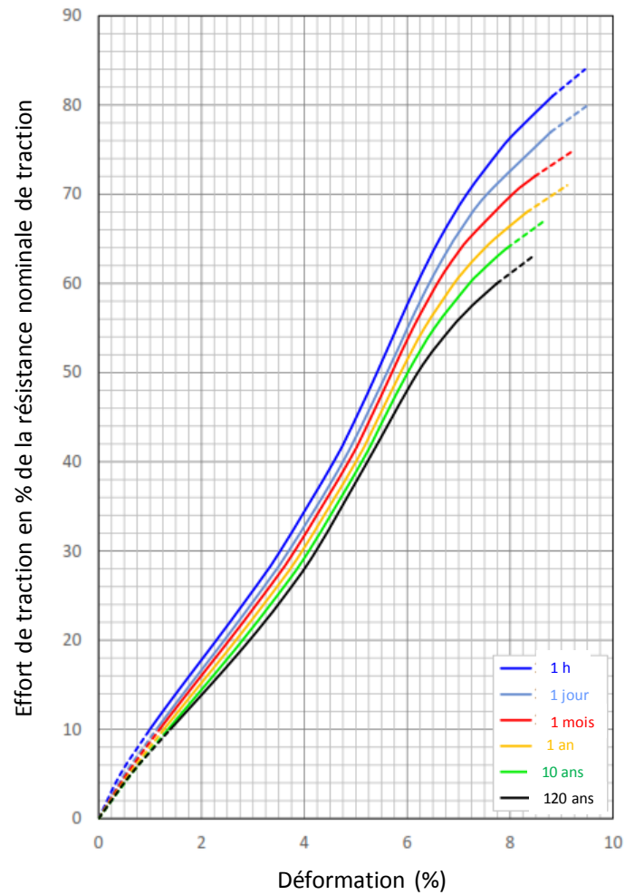
Figure 14. Courbes isochrones de la géogridde de renforcement (température de référence 20°C)
